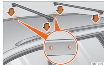
Fig. 162 Leon Sportourer ST: puntos de fijación de las barras longitudinales para el portaequipajes del techo.
