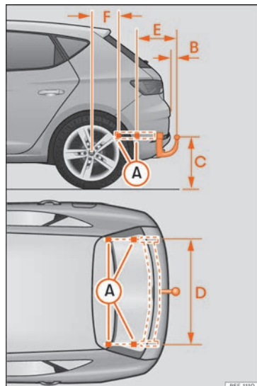
Fig. 307 Cotas y puntos de fijación para el montaje posterior de un dispositivo de remolque.
