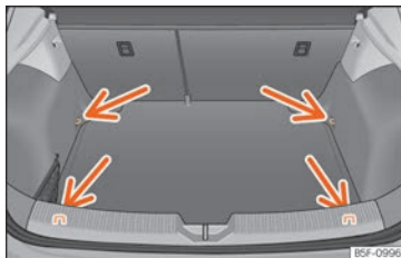
Fig. 149 En el maletero: argollas de amarre (modelo Leon excepto versiones con rueda de recambio de dotación y CNG).
