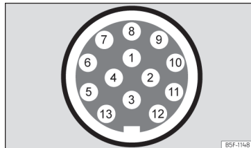
Fig. 297 Representación esquemática: asignación de los pines de la toma de corriente para remolque.
