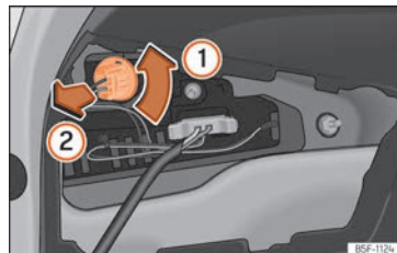
Fig. 68 Desmontar el portalámparas.
