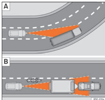
Fig. 279 [A] Vehículo en una curva. [B] Motociclista circulando por delante fuera del radio de acción del sensor de radar.
